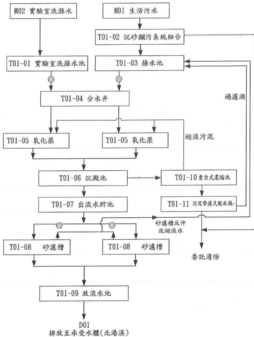
廢(污)水產生與水污染防治措施流向示意圖
